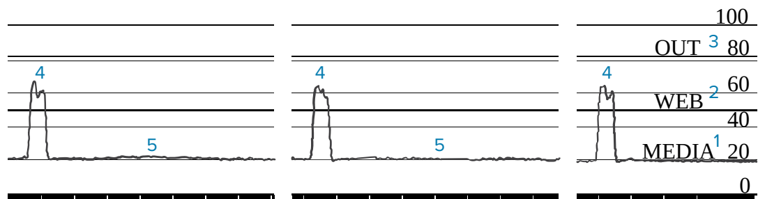
Рисунок 10 Профиль датчика (носитель с интервалами)
