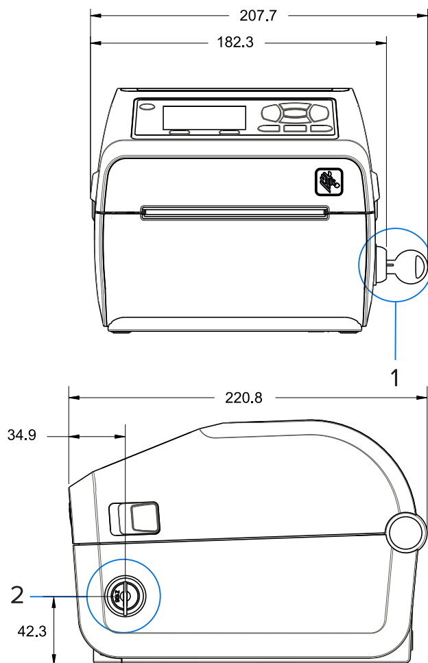
Рисунок 19 Принтер ZD621 для прямой термопечати (только для моделей, предназначенных для медицинских учреждений) с запирающимся отсеком для носителя — размеры
