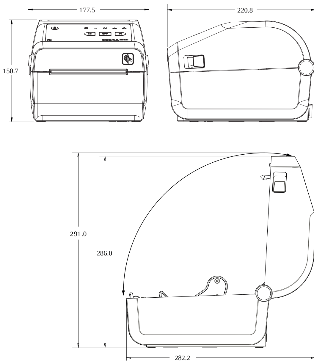
Рисунок 14 Модели принтеров ZD421/ZD621 для прямой термопечати — размеры принтера, на который установлен дополнительный модуль отделителя этикеток
