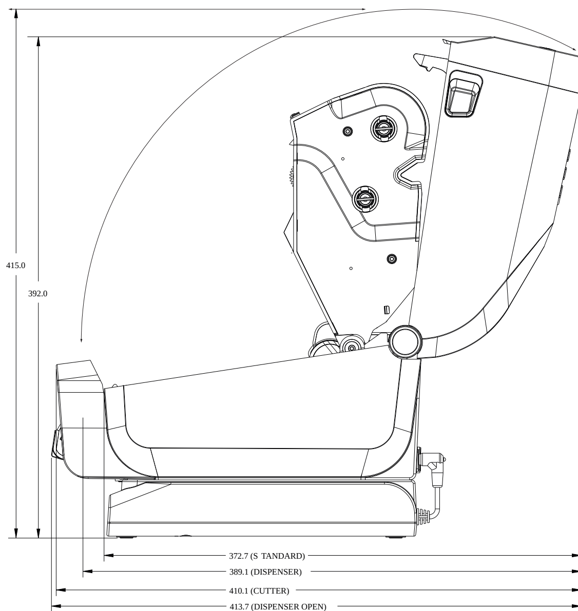
Рисунок 25 Модели принтеров ZD421/ZD621 для термопереноса — размеры открытого принтера с подключенным внешним аккумулятором
