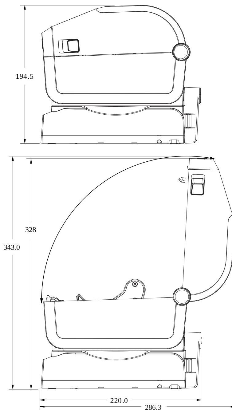
Рисунок 18 Модели принтеров ZD421/ZD621 для прямой термопечати — размеры принтера, к которому присоединены аккумуляторная база и аккумулятор
