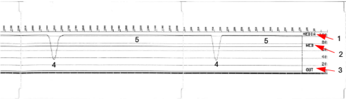
Рисунок 11 Профиль датчика (носитель для бирок с черными метками)
