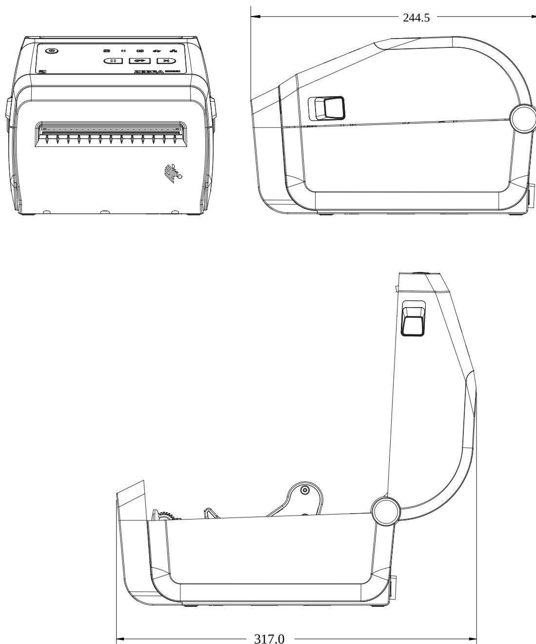
Рисунок 16 Модели принтеров ZD421/ZD621 для прямой термопечати — размеры принтера, на который установлен дополнительный модуль резака
