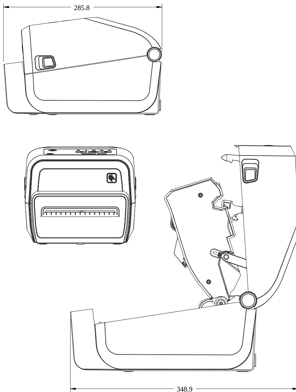
Рисунок 33 Модели принтера ZD421C (с картриджем с лентой для термопереноса) — размеры принтера с установленным дополнительным модулем резака
