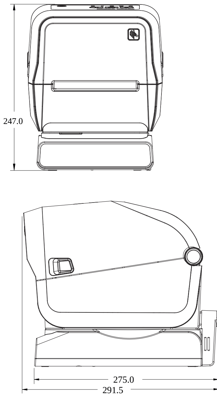
Рисунок 26 Модели принтеров ZD421/ZD621 для термопереноса — размеры принтера с присоединяемой базой с блоком питания
